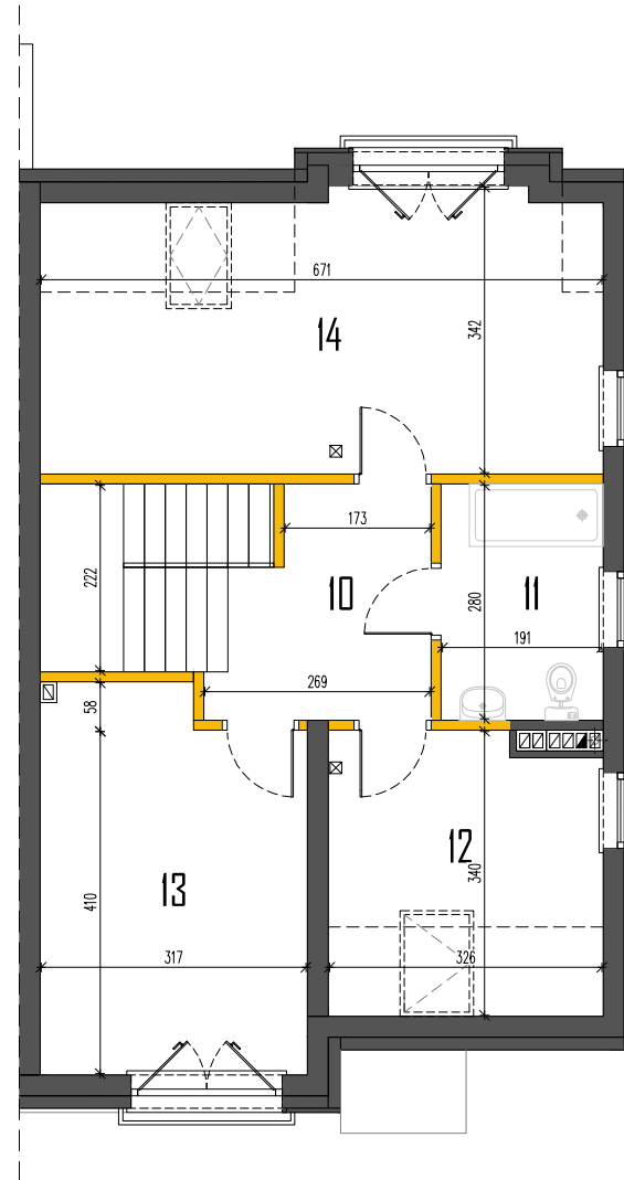
RZUT PIĘTRA
